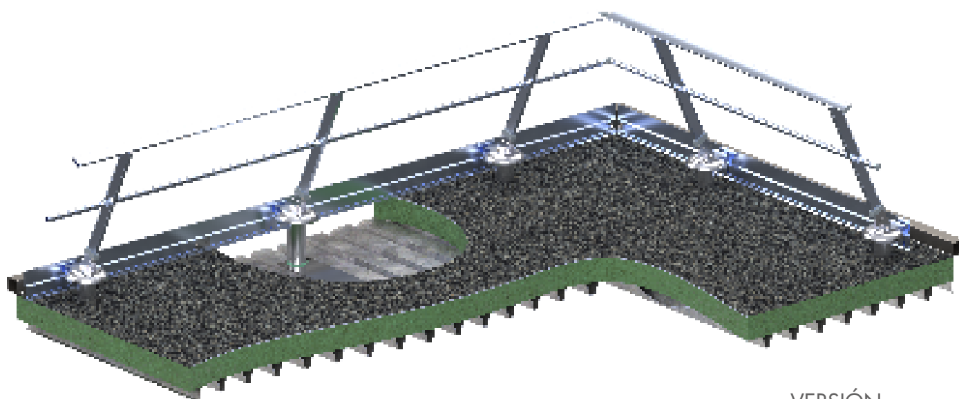
VERSIÓN INCLINADA 25°
