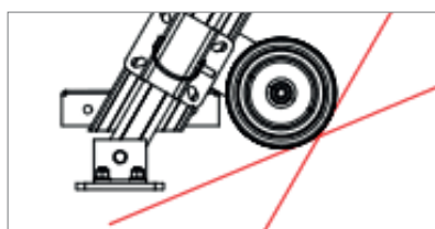
Ruedas de desplazamiento de Ø125 mm.
